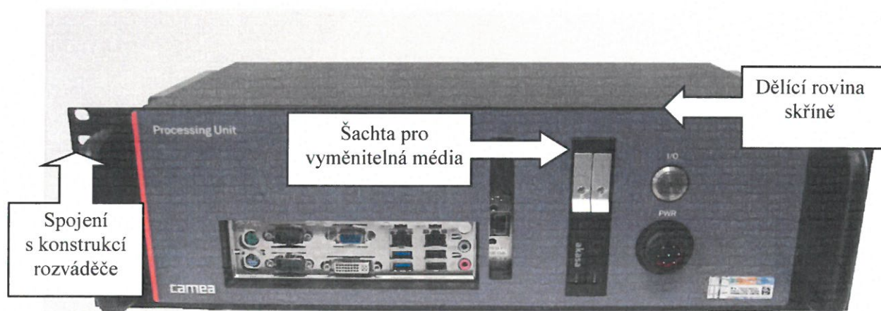
Obr. 9 Zajištění vyhodnocovací jednotky
